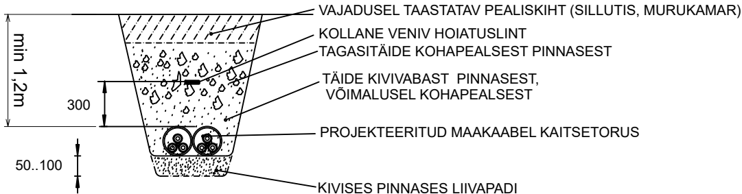
KAABLI PAIGALDUS LAHTISEL MEETODIL
