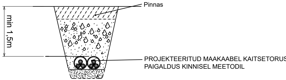
KAABLI PAIGALDUS KINNISEL MEETODIL
